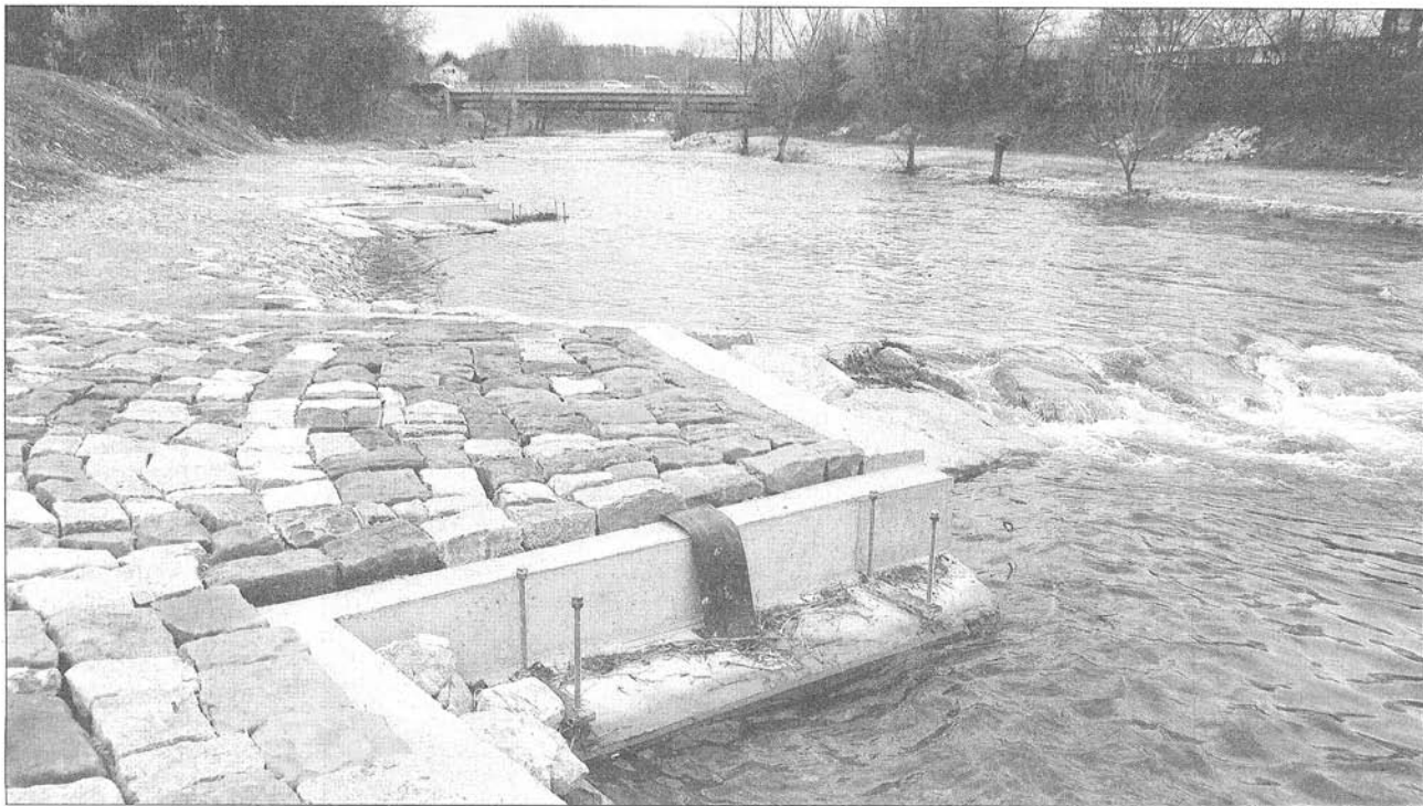
An der Wiese wurden unterhalb der Tumringer Brücke Buhnen errichtet.
